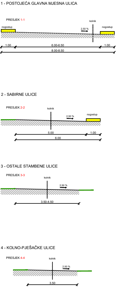
KARAKTERISTIČNI POPREČNI PRESJECI CESTA MJ 1:100
